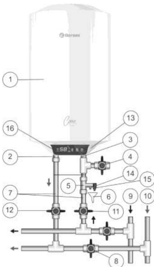
1. slika. Šema priključka električnog bojlera na vodovod
